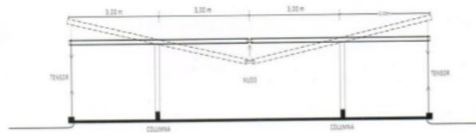
CORTE ESQUEMA ESTRUCTURAL
