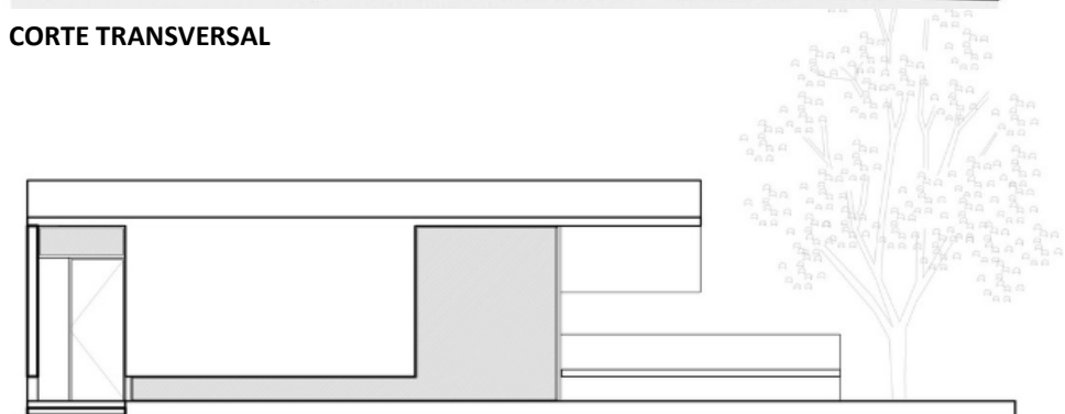
CORTE TRANSVERSAL
